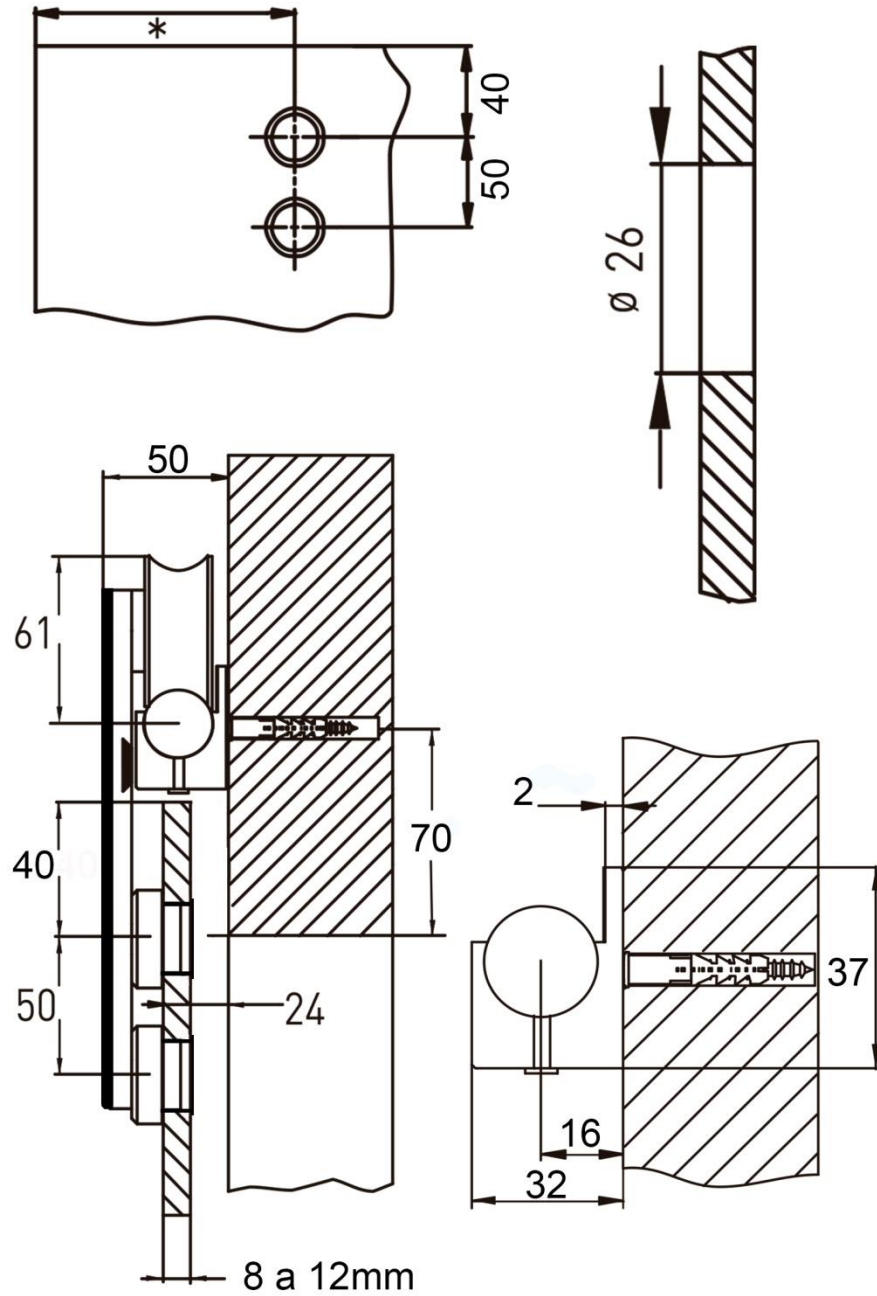
SOPORTE PERFIL PARED
